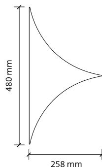
Circle link E 480 x 258 mm
