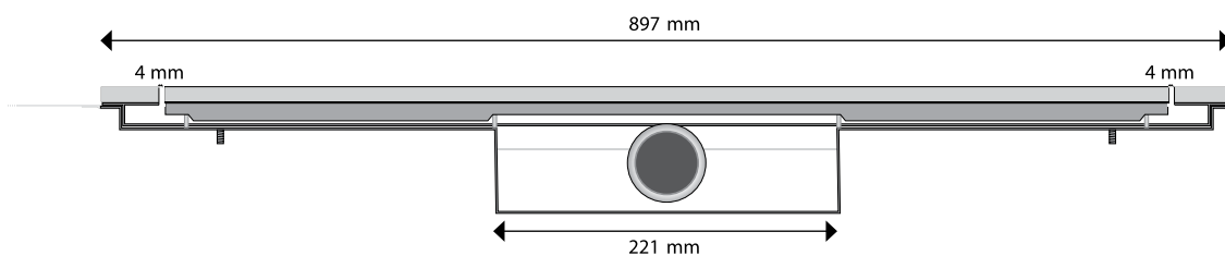
Vooranzicht Vue frontal Vorderansicht Front view (1:6,5)
